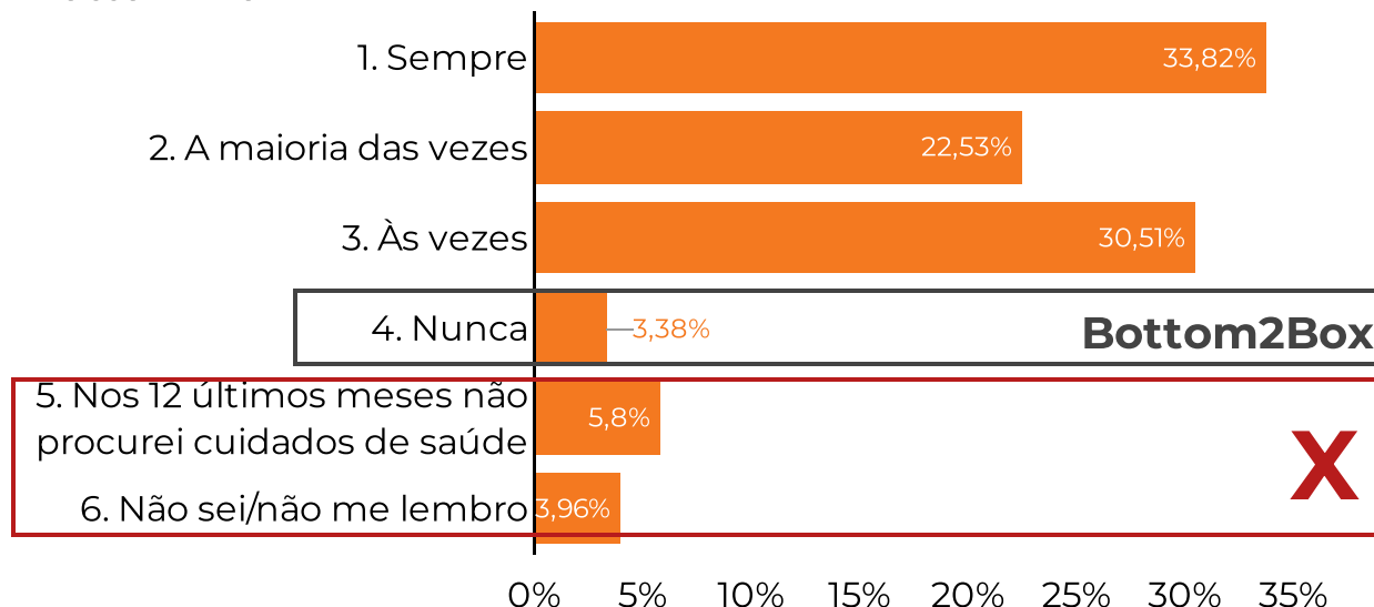
Gráfico 1: Bottom1Box
