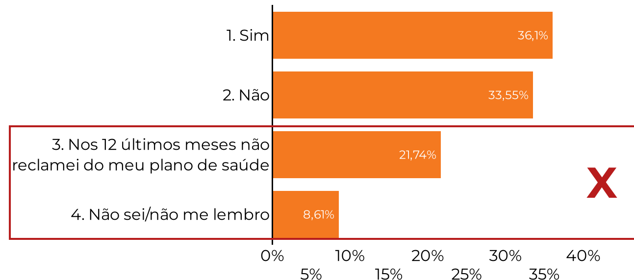
Gráfico 2: Resolutividade
